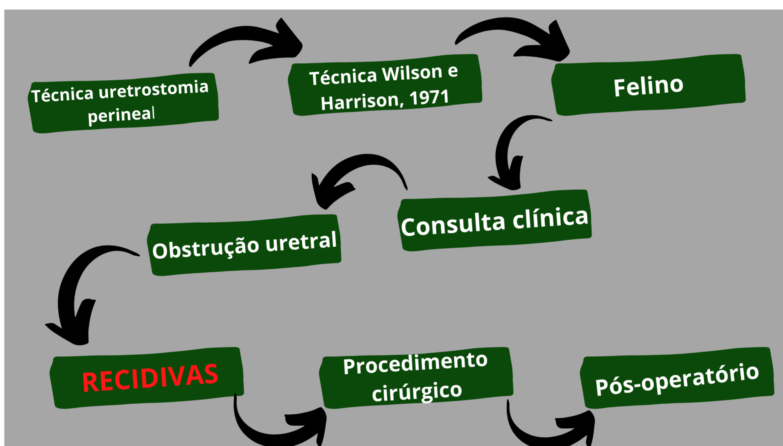
Figura 2: Metodologia.
